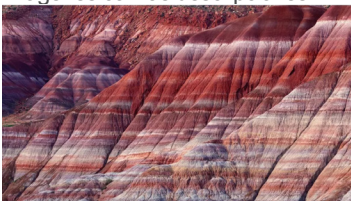
Capas sedimentarias
